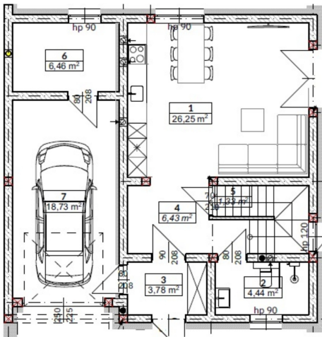
RZUT PARTERU
