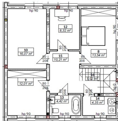
RZUT PIĘTRA
